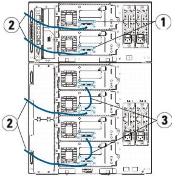
그림 5 멀티 모듈 SCSI 케이블 연결(대체 방법)
