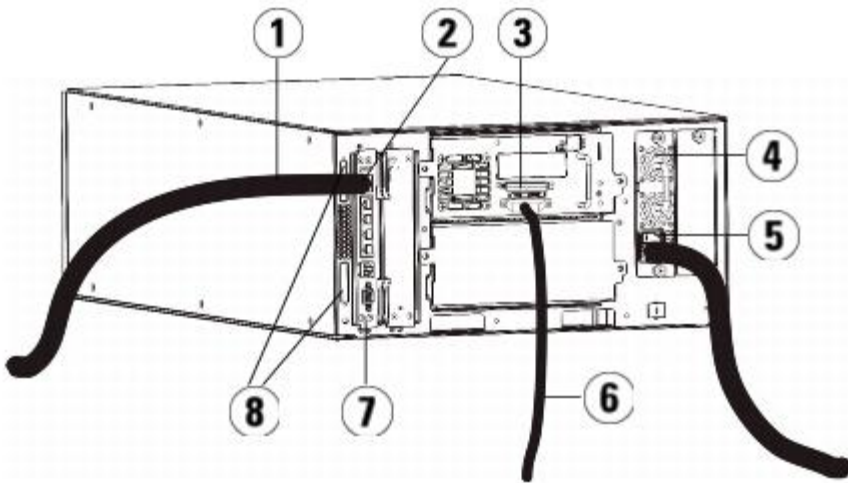
그림 3 독립형 5U 라이브러리 제어 모듈 SCSI 케이블 연결
