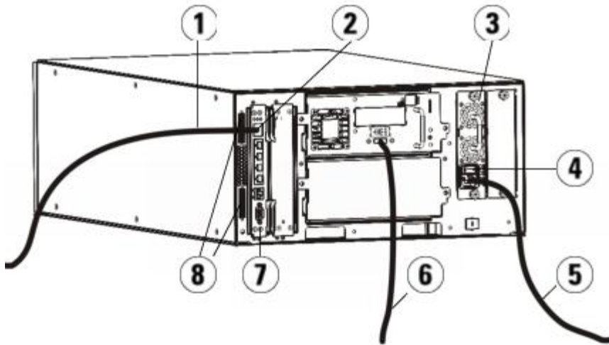
그림 10 독립형 5U 라이브러리 제어 모듈 SAS 케이블 연결
