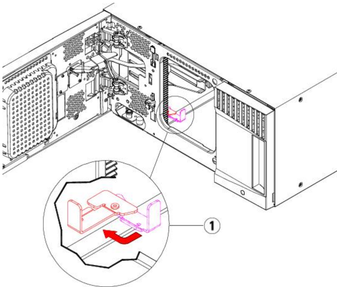
1 "파킹되지 않은" 위치의 파킹 탭
