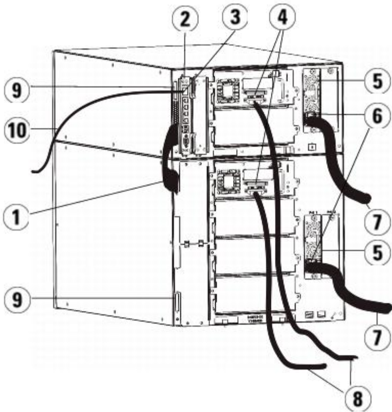
그림 4 멀티 모듈 SCSI 케이블 연결
