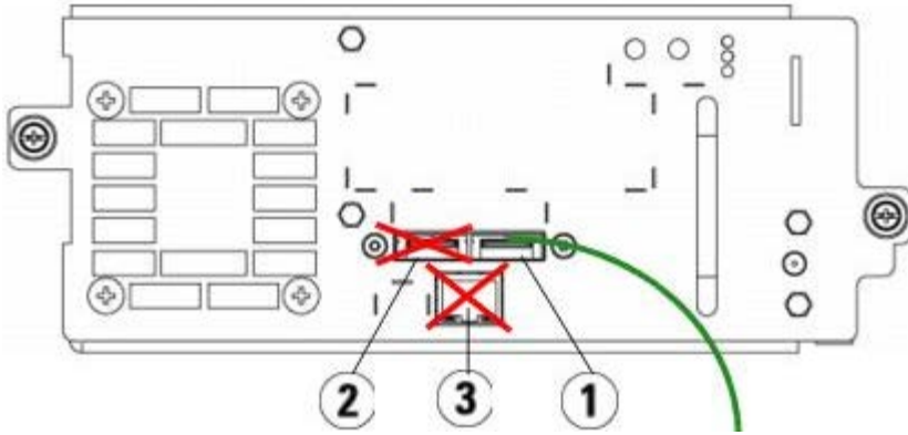
그림 2 IBM LTO-5 이중 포트 SAS 테이프 드라이브
