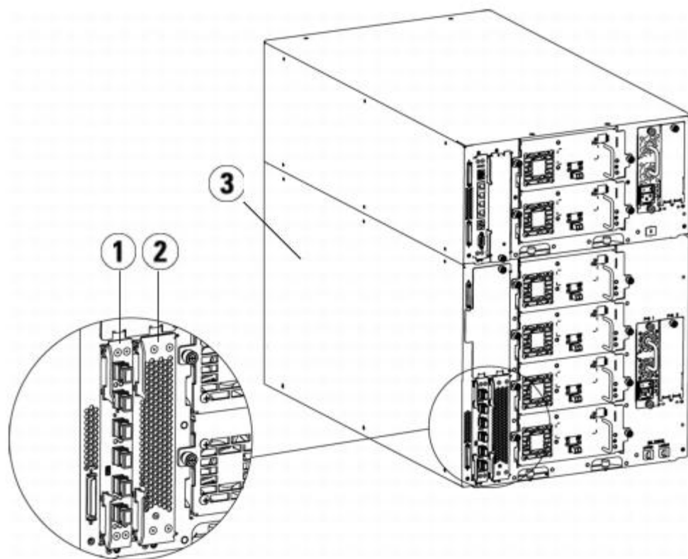
그림 21 9U 라이브러리 확장 모듈의 FC I/O 블레이드 및 팬 블레이드
