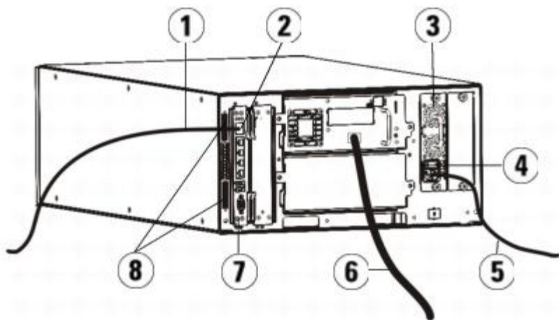
그림 6 독립형 5U 라이브러리 제어 모듈 Fibre Channel 케이블 연결
