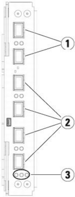
그림 9 FC I/O 블레이드
