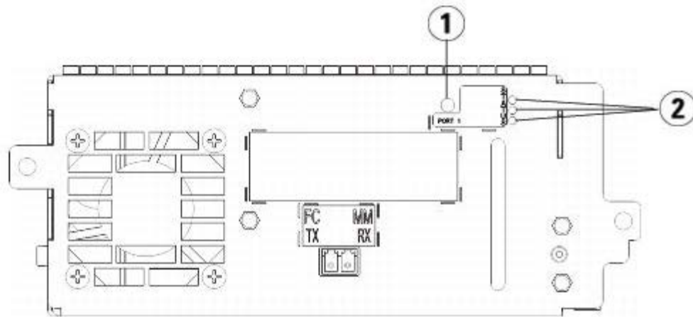
그림 1 테이프 드라이브 LED의 위치
