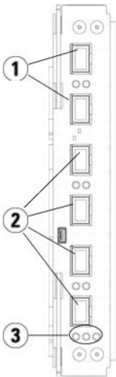
그림 8 FC I/O 블레이드
