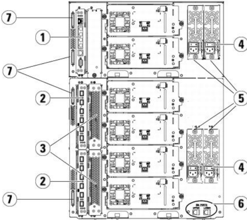
그림 6 후면 패널 구성 요소
