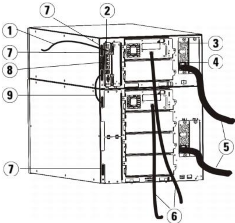
그림 7 멀티 모듈 Fibre Channel 케이블 연결
